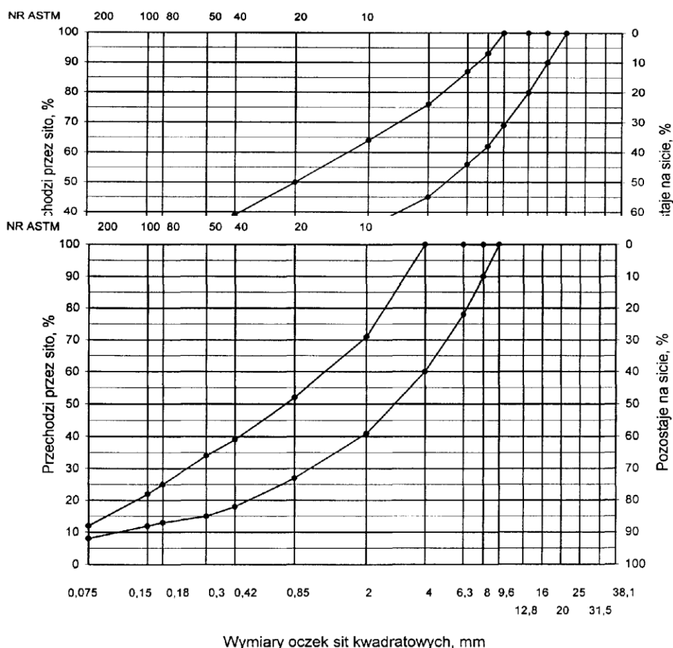
Rys. 2. Krzywe graniczne uziarnienia mieszanki mineralnej BA od 0 do 16mm, od 0 do 12,8 mm do warstwy ścieralnej nawierzchni drogi o obciążeniu w ruchu KR1 lub KR2
