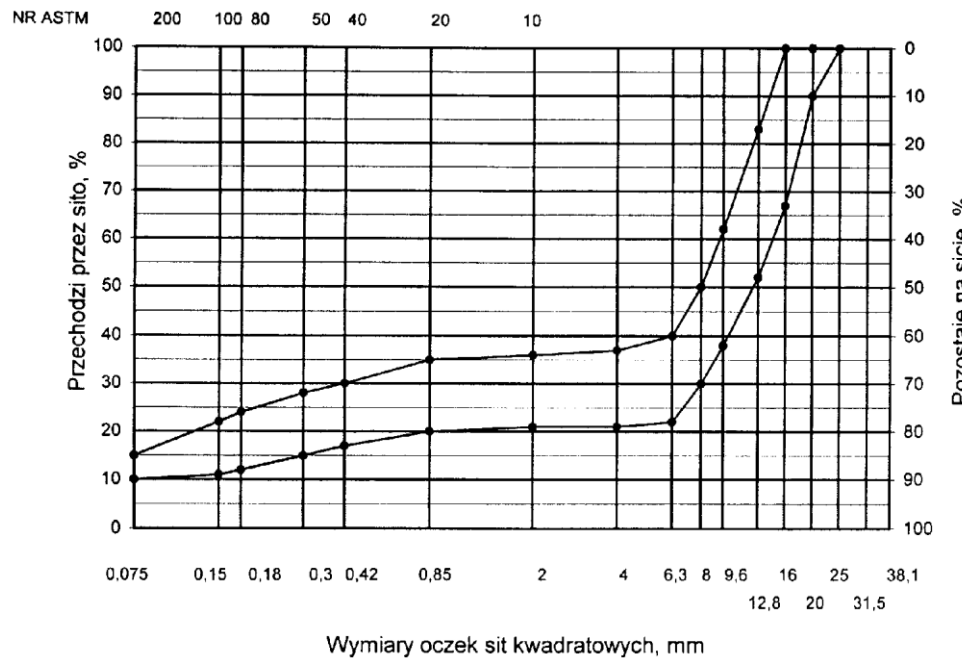
warstwy ścieralnej nawierzchni drogi o obciążeniu ruchem od KR3 do KR6
