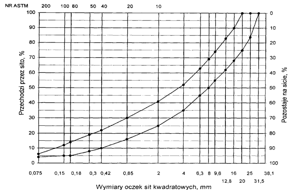
Rys. 11. Krzywe graniczne uziarnienia mieszanki mineralnej BA od 0 do 25 mm do warstwy wiążącej, wyrównawczej i wzmacniającej nawierzchni
